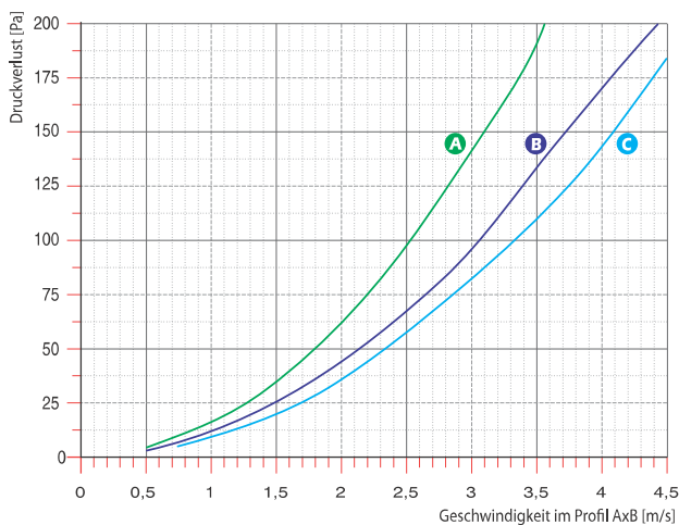
Diagramm Druckverlust [Pa]
