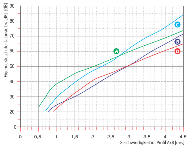
Diagramm Eigengeräusch L_w durch Luftströmungseinfluss [dB]
