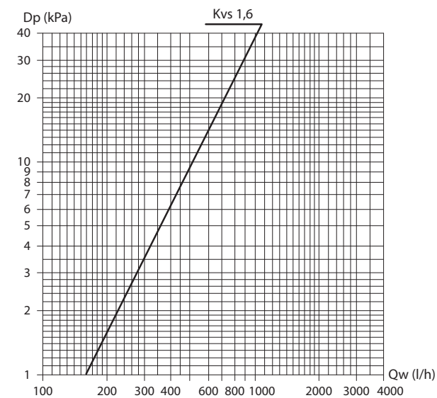
Druckverluste 3-Wege-Ventile
