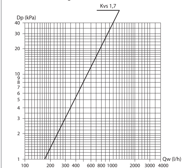
Druckverluste 2-Wege-Ventile
