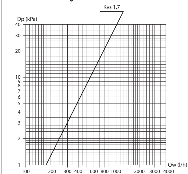
Druckverluste 2-Wege-Ventile
